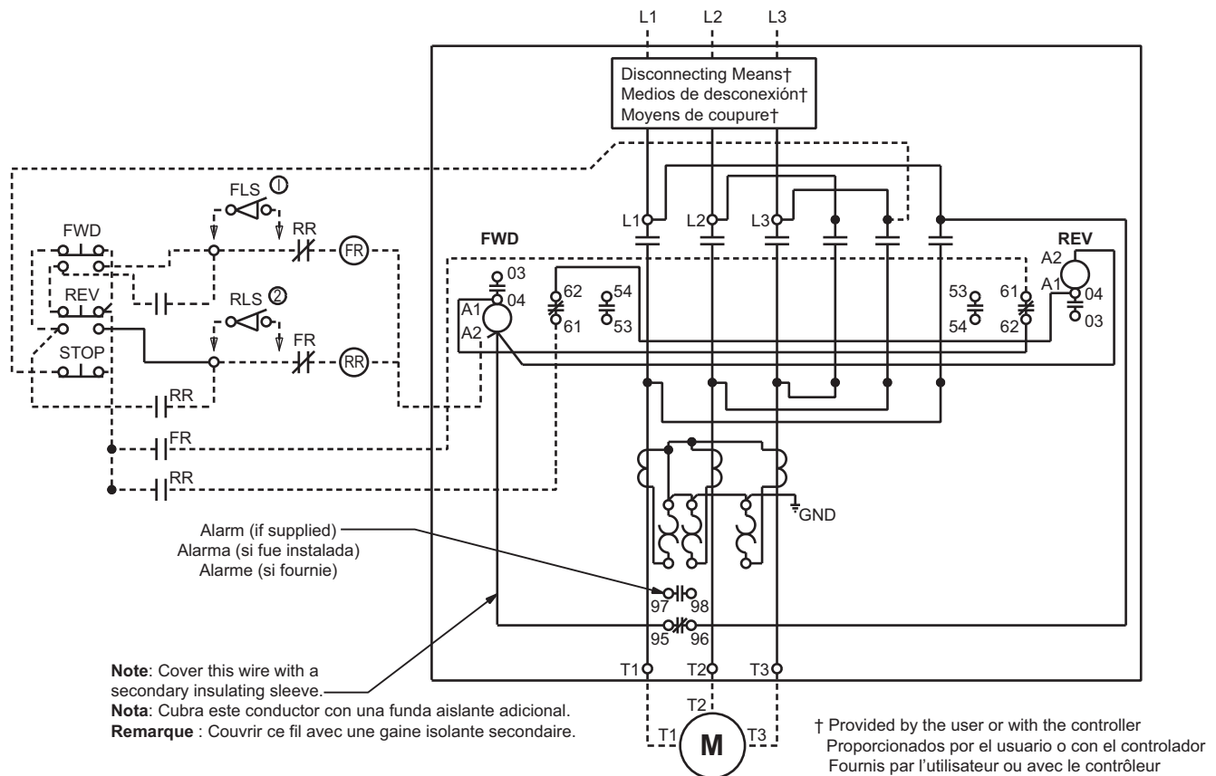
FIG. 5 : NEMA Size 5–7, Common Control, With Interposing Relay NEMA tamaños 5 a 7, control común con relevador de interposición NEMA tailles 5 à 7, contrôle commun, avec relais d'interposition
