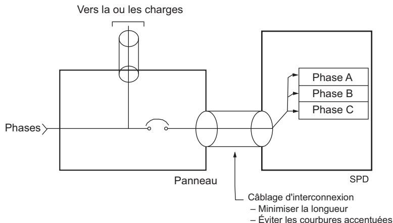
Figure 3: Câblage du SPD pour les configurations en triangle
