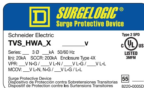
Figure 1 : Exemple de plaque signalétique du SPD
