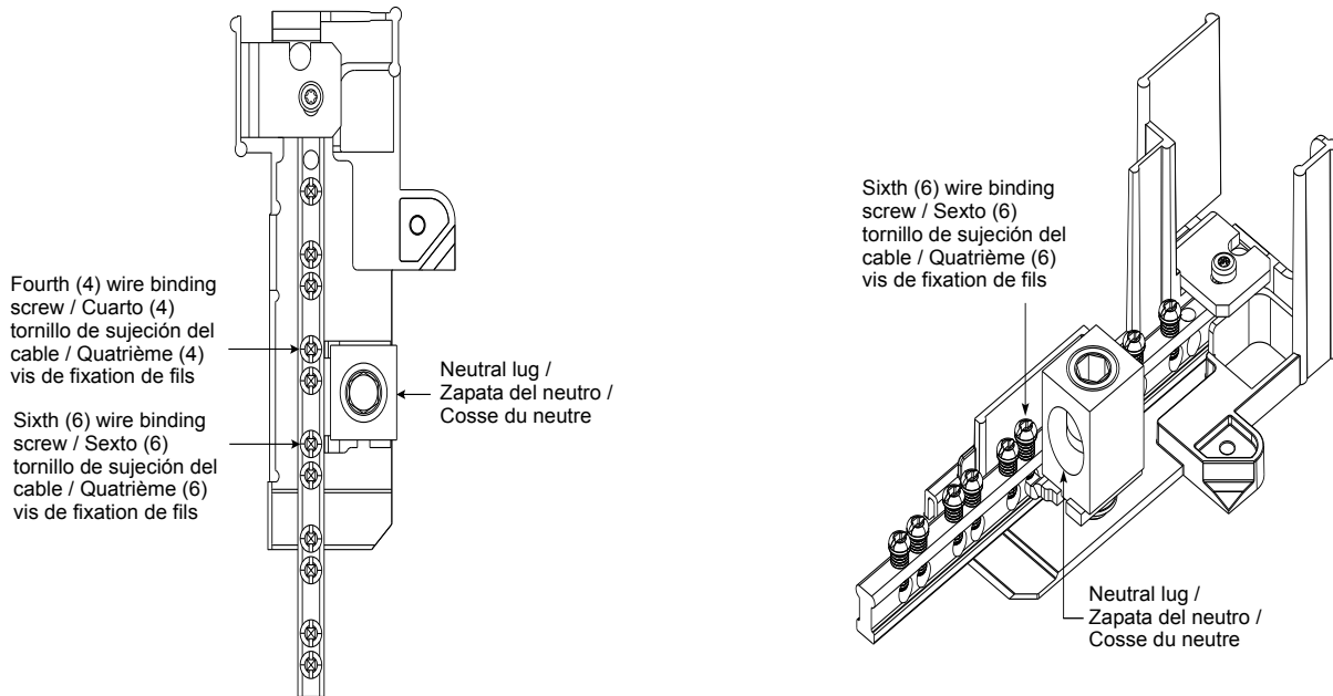
Figure / Figura / Figure 1 : Installing the Neutral Lug Kit into the Homeline Load Center / Instalación del accesorio de la zapata del neutro en el centro de carga Homeline / Installation du kit de cosse du neutre dans le centre de distribution Homeline
