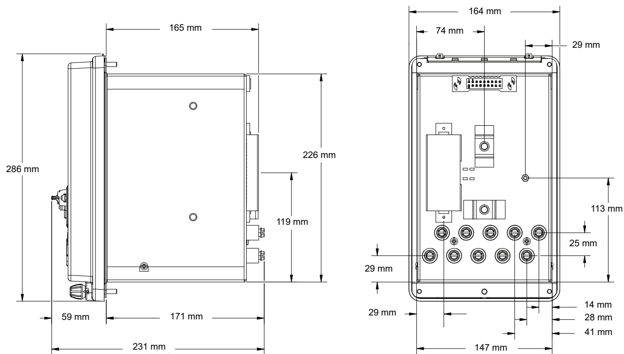
Boîtier de tableau FT-21 avec câble de dérivation
