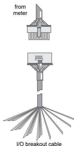
I/O breakout cable
