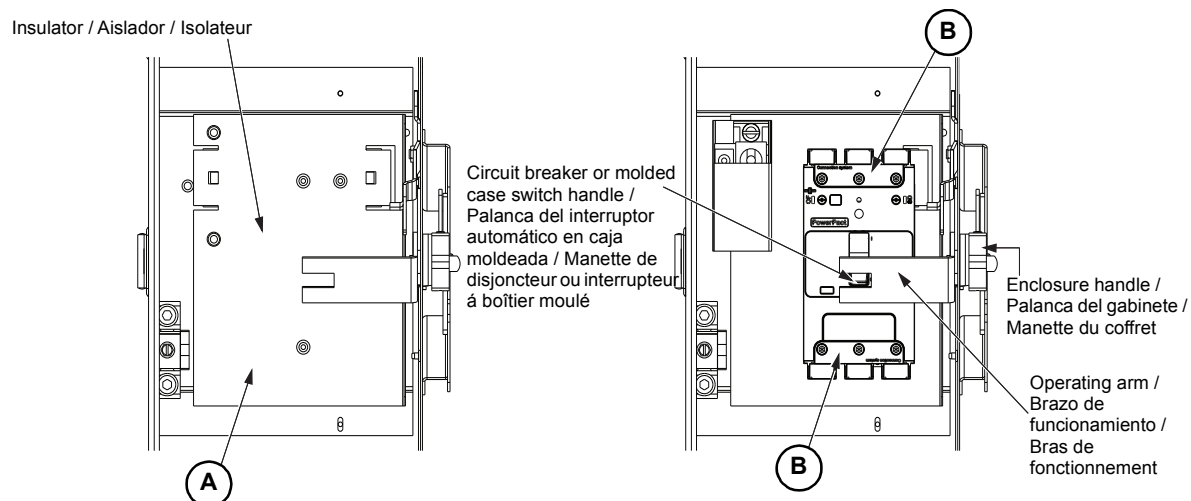
Figure / Figura / Figure 1 : Installing the Circuit Breaker or Molded Case Switch / Instalación del interruptor automático o interruptor en caja moldeada / Installation du disjoncteur ou de l'interrupteur à boîtier moulé
