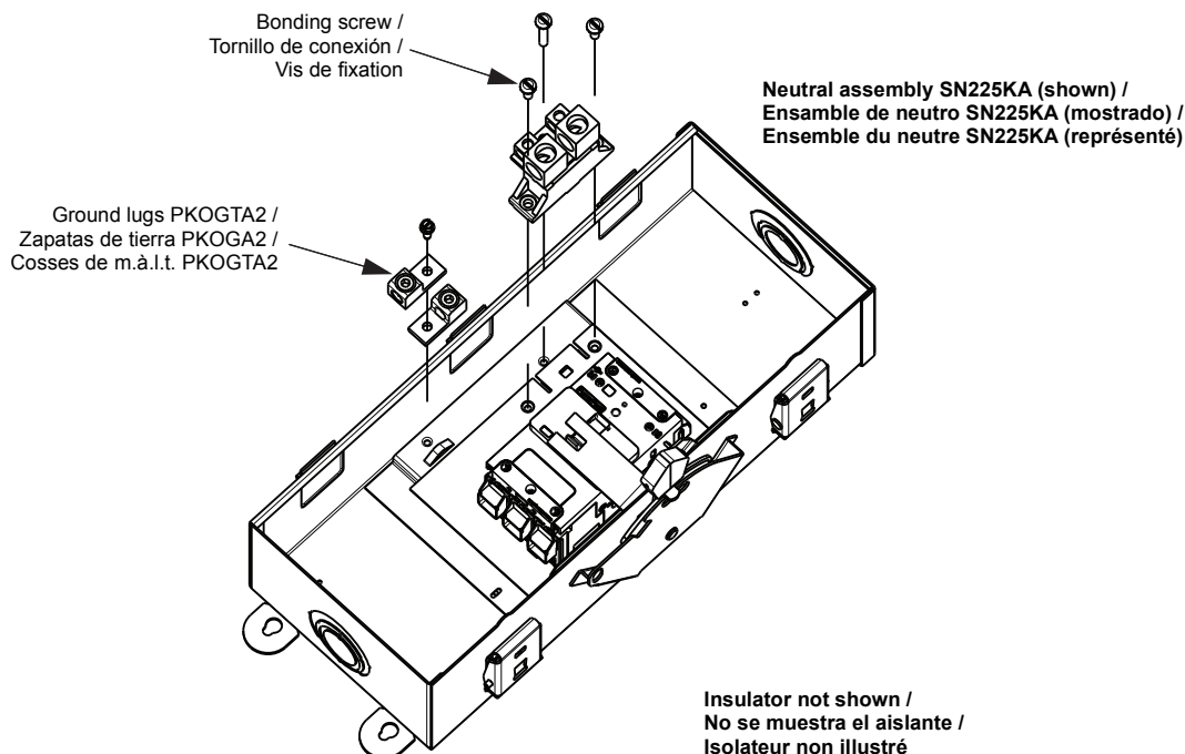
Figure / Figura / Figure 2 : Installing the Neutral Assembly / Instalación del ensamble del neutro / Installation de l'ensemble du neutre
