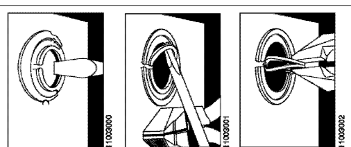
Figure / Figura / Figure 1 : Removing Knockouts / Extracción de los discos desprendibles / Retrait des débouchures
