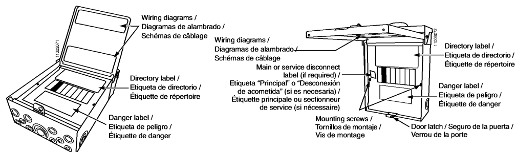
Figure / Figura / Figure 5 : Label Application / Cómo colocar las etiquetas / Application des étiquettes
