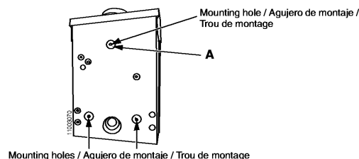
Figure / Figura / Figure 2 : Mounting the Box / Cómo montar la caja / Montage du boîtier
