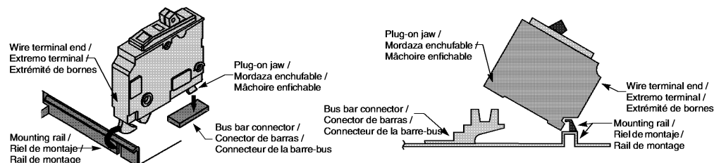
Figure / Figura / Figure 4 : Branch Circuit Breakers / Interruptores automáticos derivados / Disjoncteurs de dérivation
