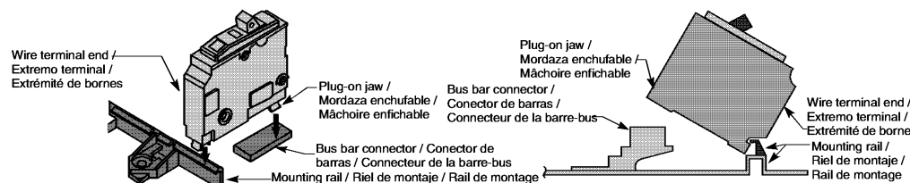
Figure / Figura / Figure 3 : QO® or Homeline® Branch Circuit Breakers / Interruptores automáticos derivados QO® o Homeline® / Disjoncteurs de dérivation QO® ou Homeline®
